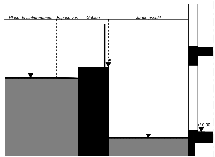
COUPE A-A
